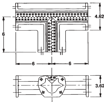
VFH-T 12" x 6" tee
